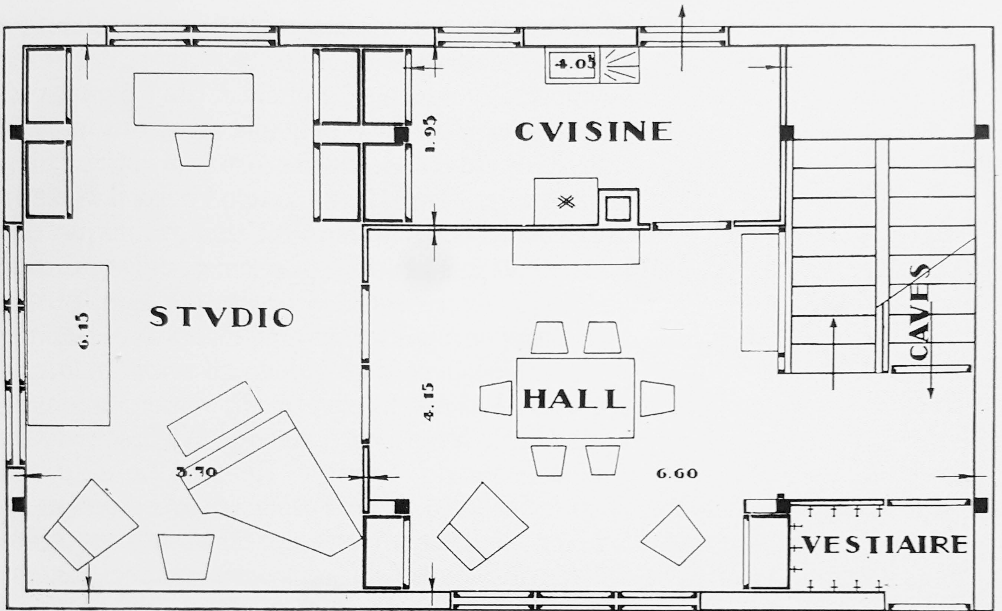
REZ-DE-CHAUSSÉE TYPE B.
